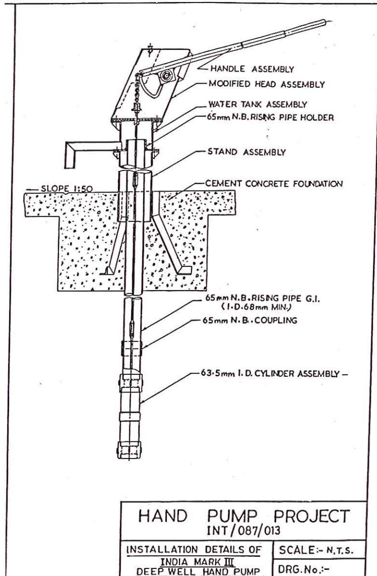
Konstruktionsritning till India Mark II
